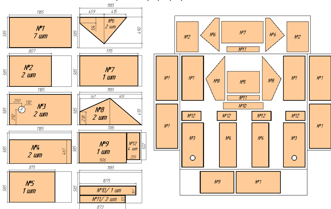
Рисунок 7 – Карта раскроя утеплителя
